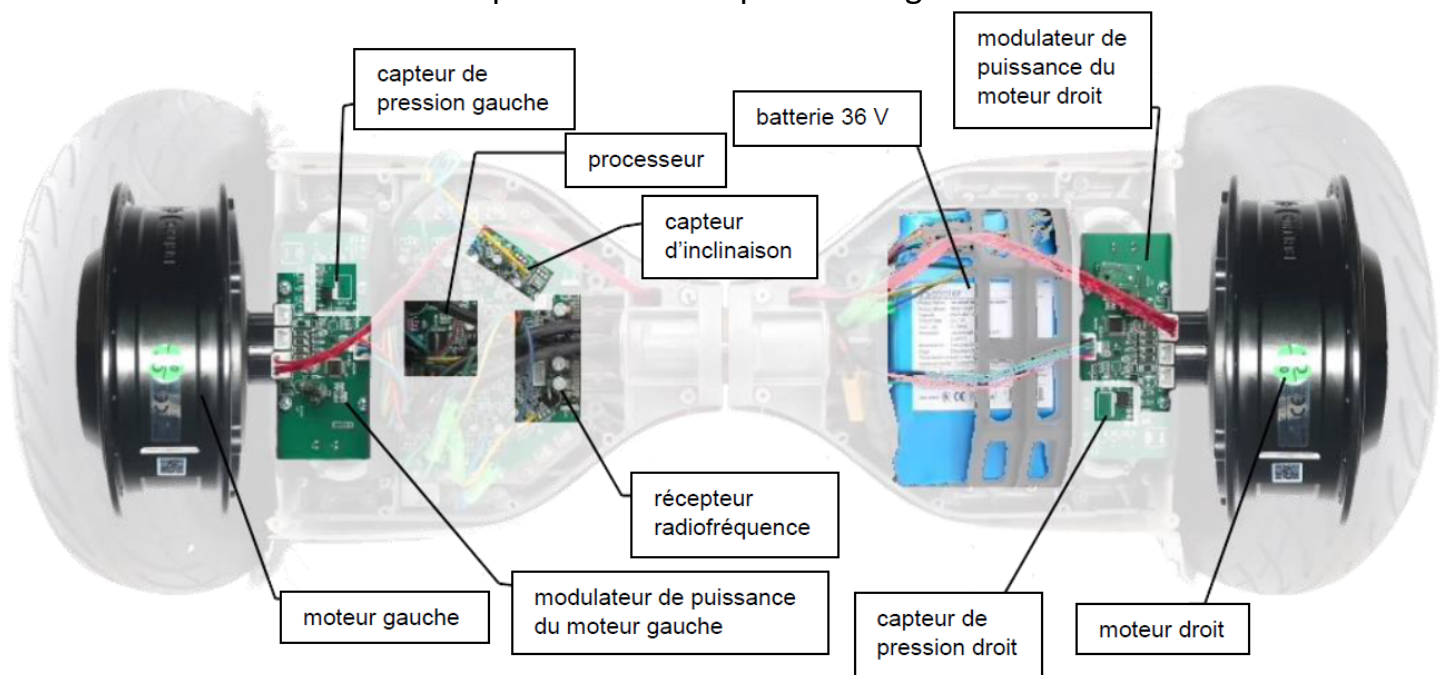
Figure 2 : vue interne de l'overboard Xenox
